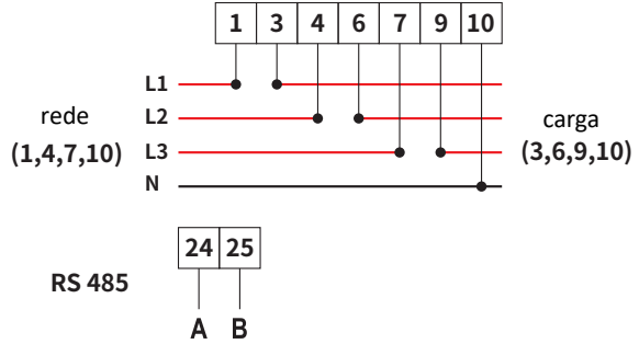
Figura 7.28 Medidor CHINT
