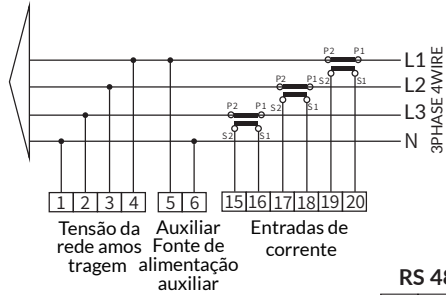
Figura 7.5 Medidor Eastron
